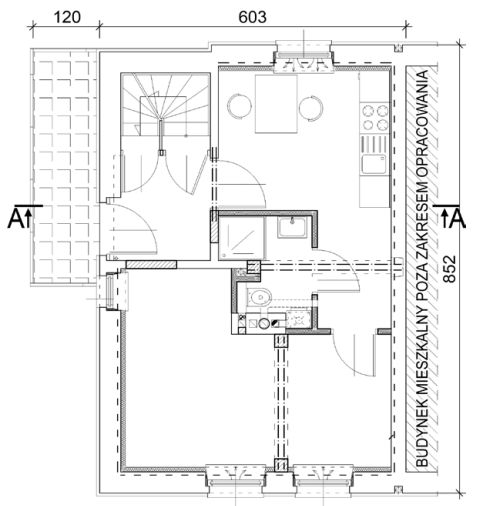
RZUT PARTERU
