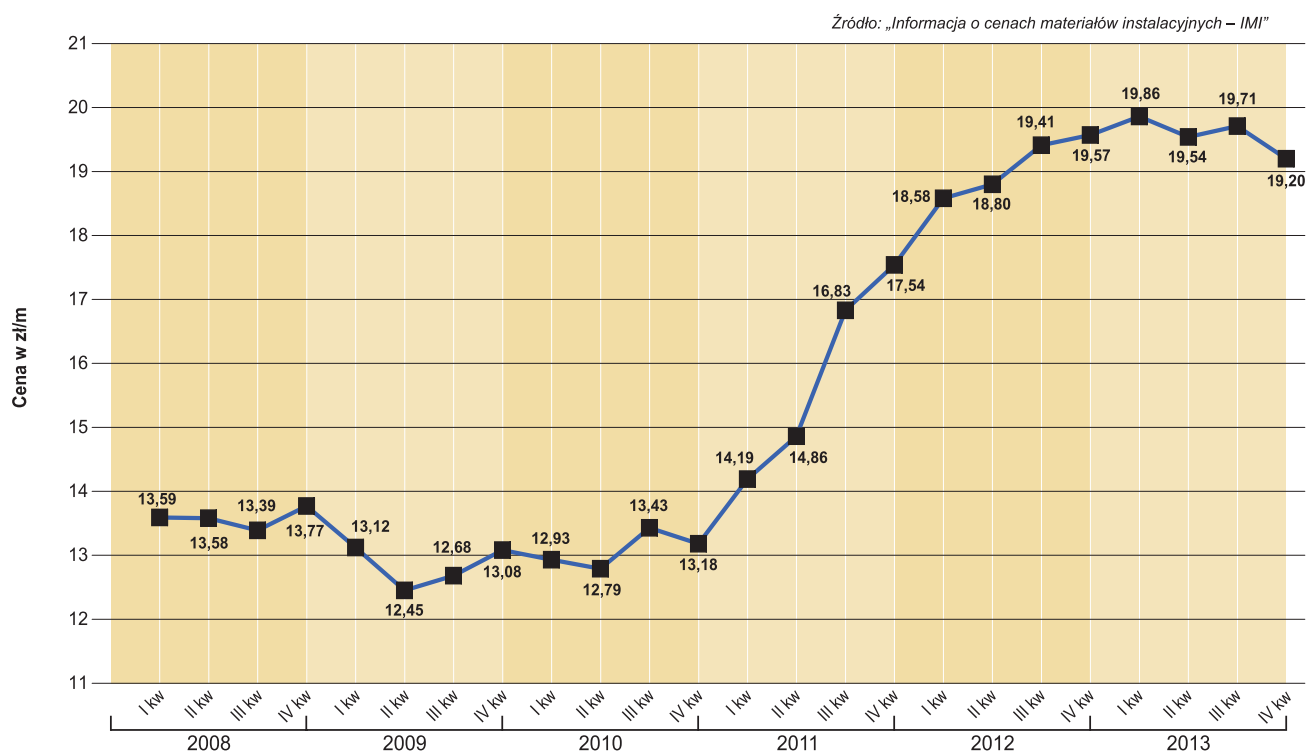
Wykres 18. Ceny rur miedzianych ø 15 mm – w latach 2008-2013
